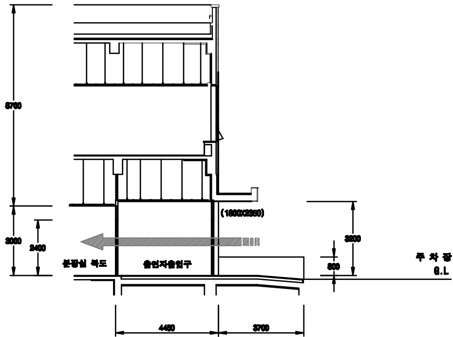
콘서트홀 악기 / 장치반 입구 단면도
