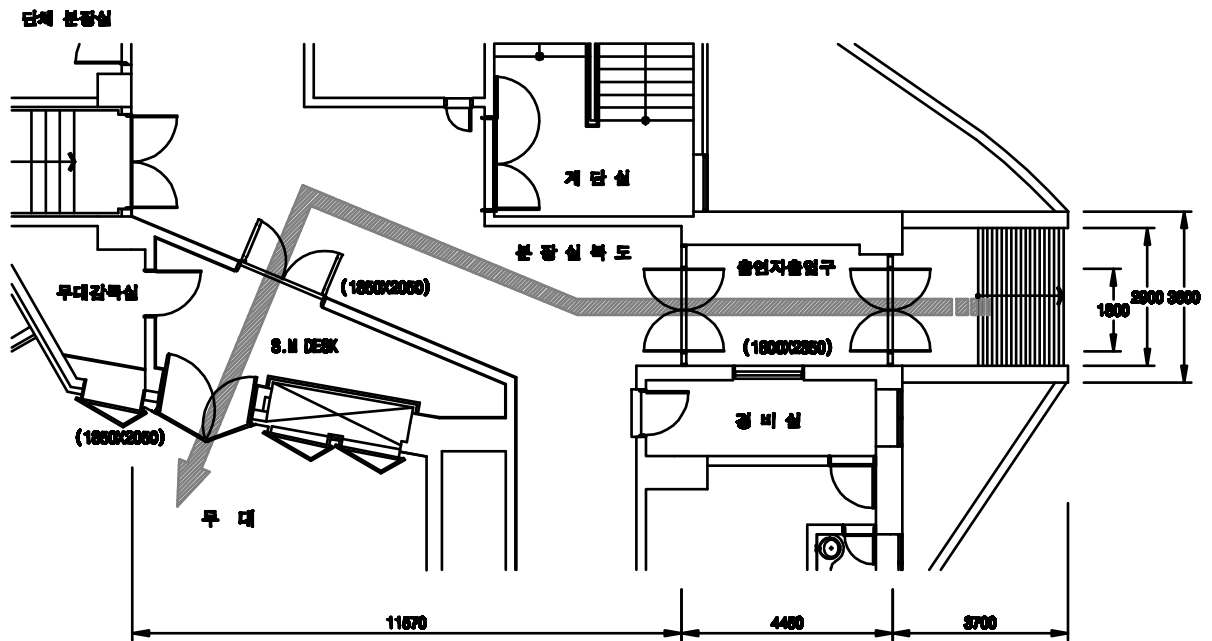
콘서트홀 악기 / 장치반 입구 평면도
