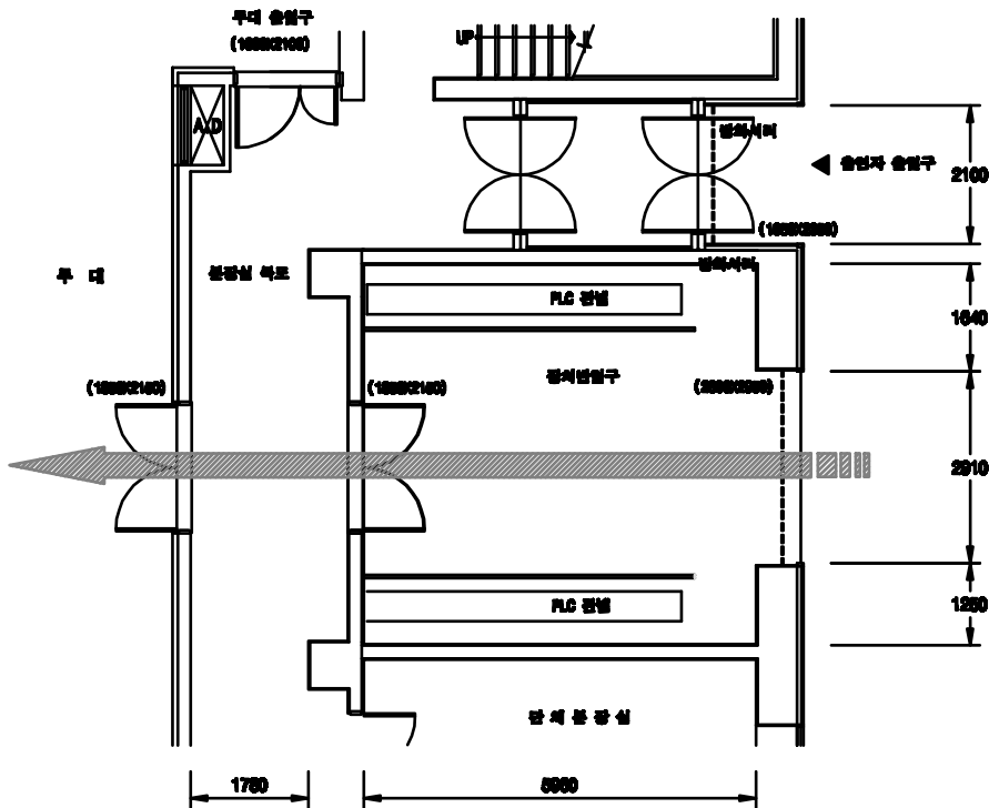
양상발전소 2층 장치반 입구 평면도
