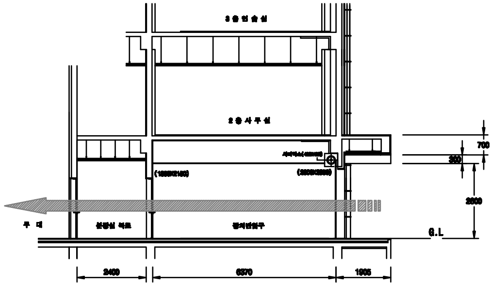
양상발전소 2층 장치반 입구 단면도
